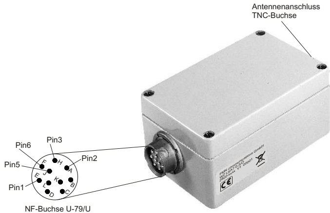
Abbildung 3-2: Bezeichnung der 6-poligen Anwenderschnittstelle (IP65 Gehäuse)
