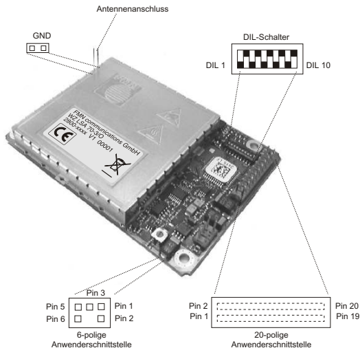
Abbildung 3-1: Bezeichnung der Funktionselemente (Platinenversion)
